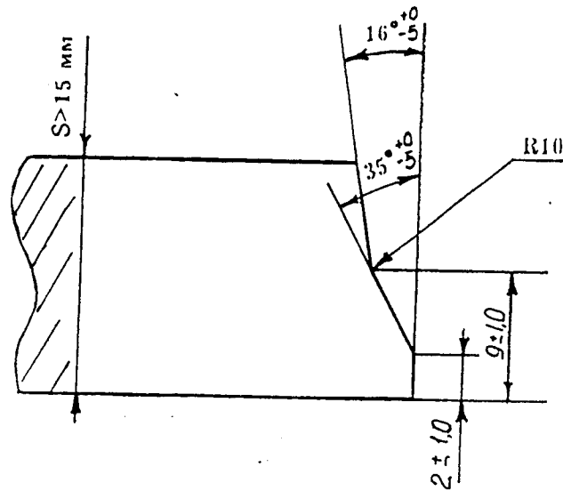
Рис. 1 Разделка кромок торцов трубы.
